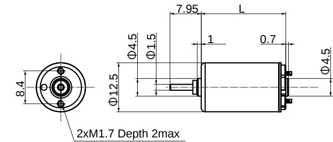
寸法図 / Dimension
