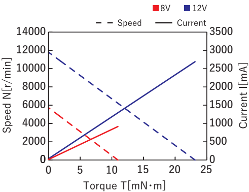
特性図 / T-N-I curve
