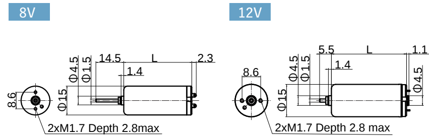
寸法図 / Dimension
